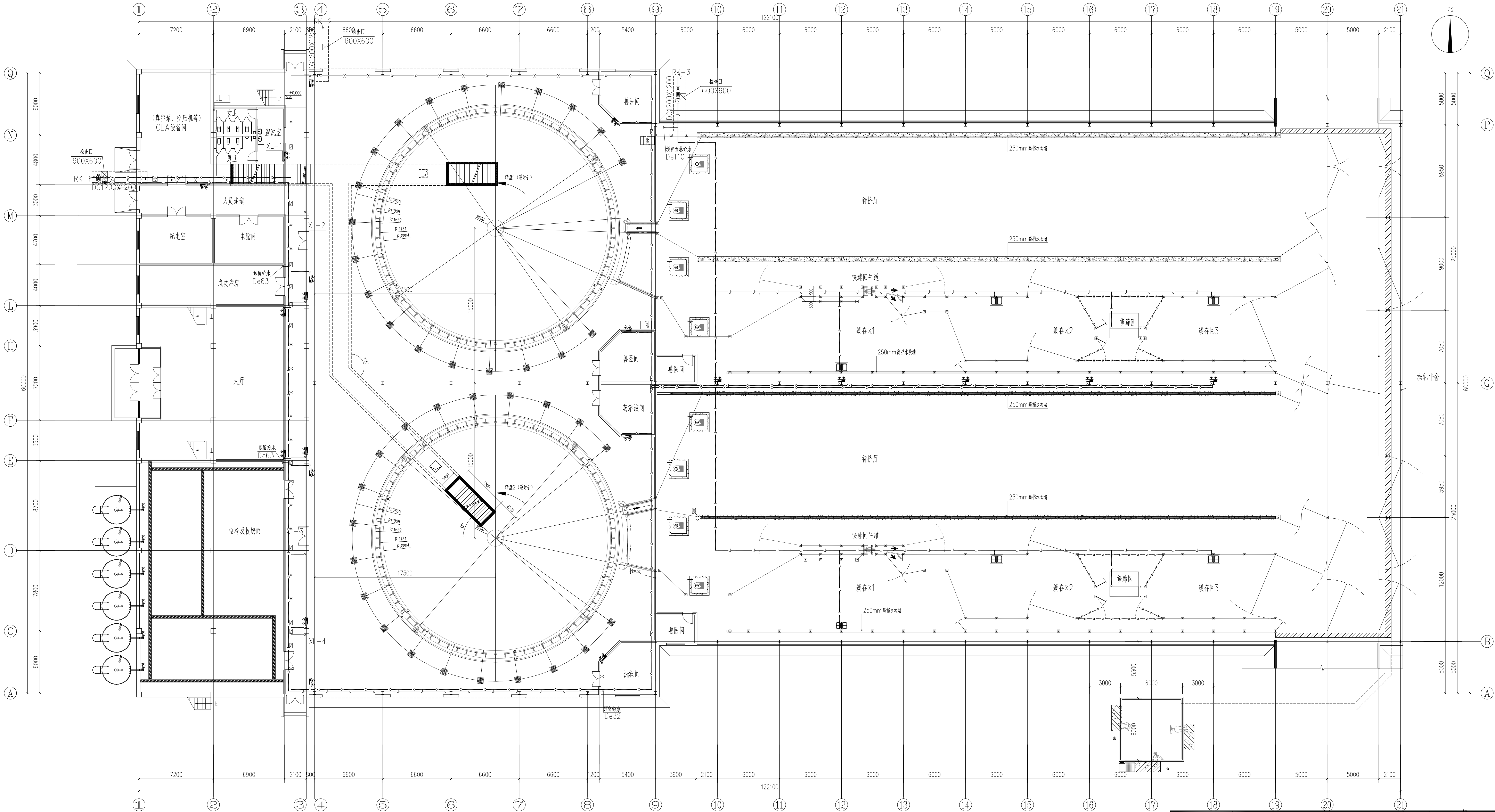
一层给水、消防平面图 1:150
